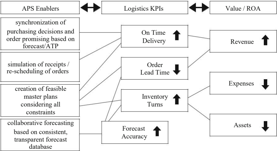
Fig. 15.8 Enabler-KPI-value network
